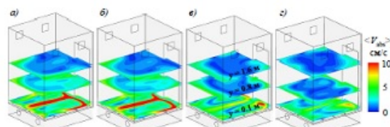
Рис. 3. Поля модуля скорости в трех горизонтальных сечениях при разных коэффициентах гидравлического сопротивления ( \zeta ): а) 0, б) 1.25, в) 25, г) 100
